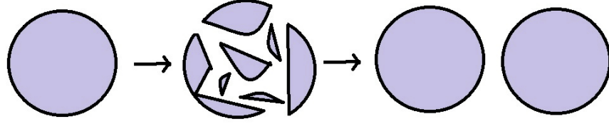
Figura 4.3: Ilustración del teorema de Banach-Tarski. Si se admite el principio de elección, se puede seccionar una bola en diversos trozos y luego ensamblarlos para construir dos bolas iguales a la inicial.
