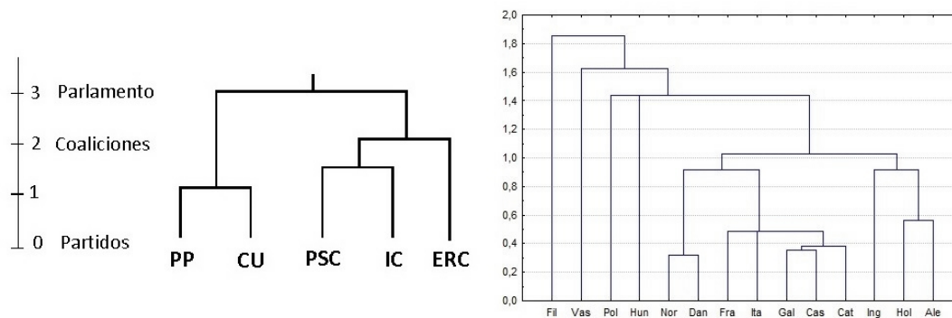
Figura 6.1: Representación de cinco partidos políticos, visualizando mediante un dendograma de la jerarquía indexada. A la derecha dendograma de 14 idiomas europeos según la semejanza entre algunas palabras comunes.
