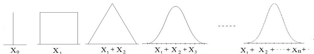
Figura 3.2: El teorema central del límite es un resultado estadístico importante que ilustra la sucesión 0, 1, \dots, n, \dots, \omega . El ordinal \omega correspondería a la distribución normal.
