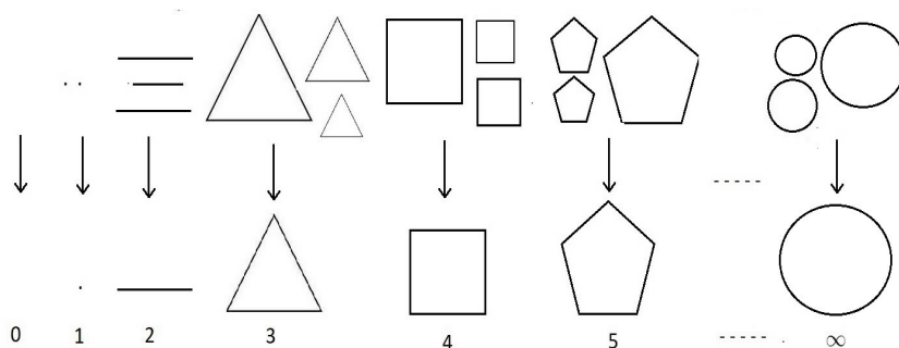
Figura 5.1: Aplicando el principio de elección, podemos seleccionar una clase de conjuntos formada por figuras de un punto, de dos vértices, de tres, de cuatro, de cinco, etc., de modo que tengamos una sola figura para cada colección de polígonos. El límite de estos polígonos se identifica con una circunferencia (infinitos vértices), aunque no da lugar a la circunferencia completa.
